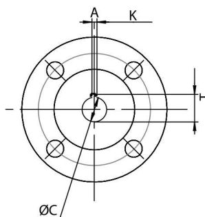
Присоединительный фланец
