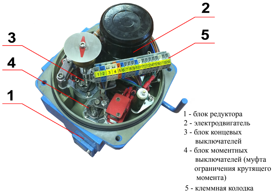
Рис. 2. Основные элементы конструкции электропривода тип QT
